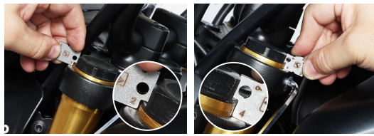
Protrusion : 2 mm
