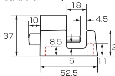
側面図 (OPEN)
