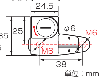
上面図 (LOCK)
