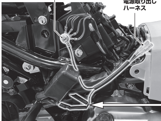
フレームアースポイント
