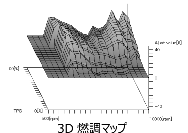
3D 燃調マップ
